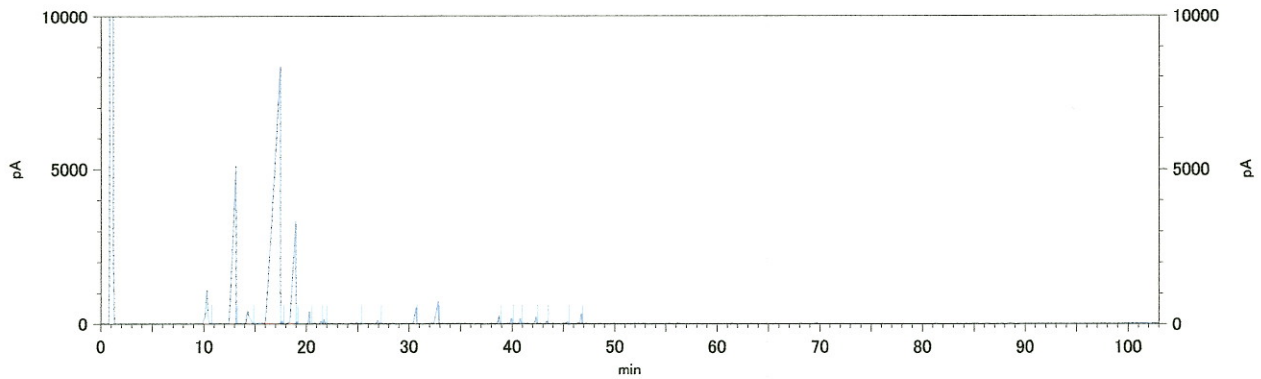
【図1. 広島レモンオイルのGC分析グラフ】
